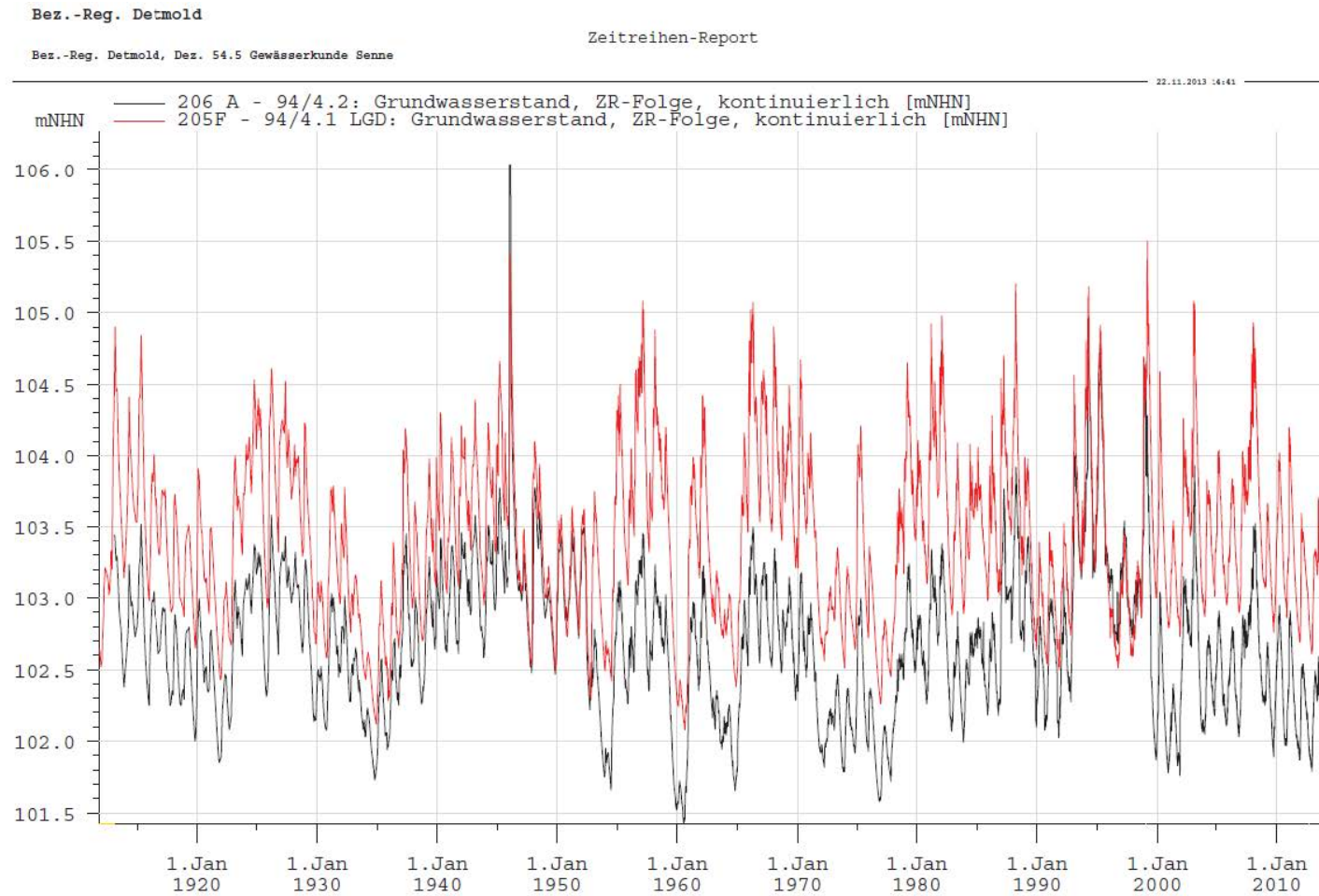
Abb. 5: Ganglinien vom gesamten Beobachtungszeitraum der Messstellen 205 Flach und 206 Tief
