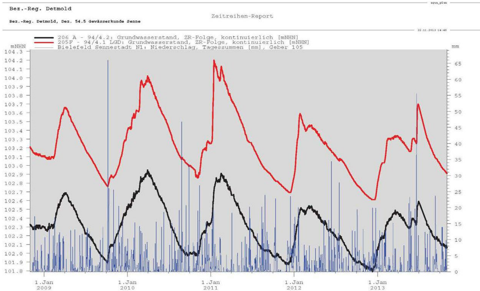
Abbildung 7 Ganglinien der WWJ 2009 bis 2013 der Mess-Stellen 205 Flach und 206 Tief (Tageswerte) zusammen mit den Tagessummen des Niederschlages der Wetterstation Sennestadt
