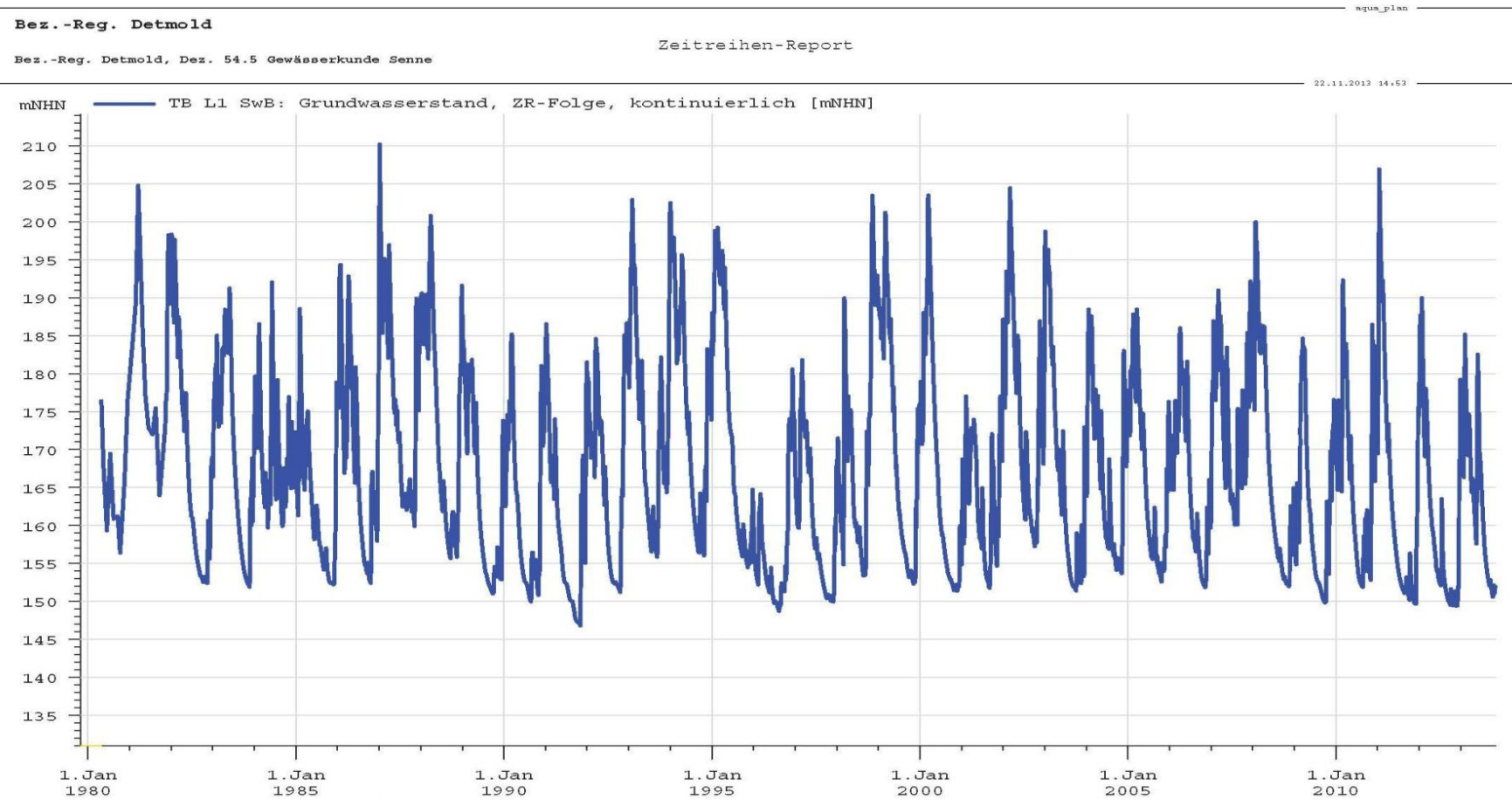
Abbildung 8 Grundwasser-Ganglinie der Mess-Stelle TB L 1 vom Beobachtungszeitraum 1980 bis 2013. Lage: Teutoburger Wald im Bereich Oerlinghausen
