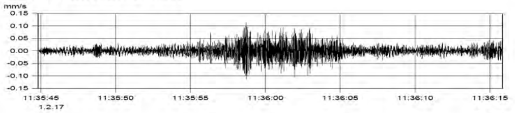
MP2.1 (Kanal_002) v(max) = 0.114 mm/s
