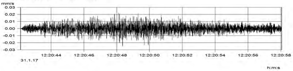
MP1 (Kanal_001) v(max) = 0.025 mm/s
