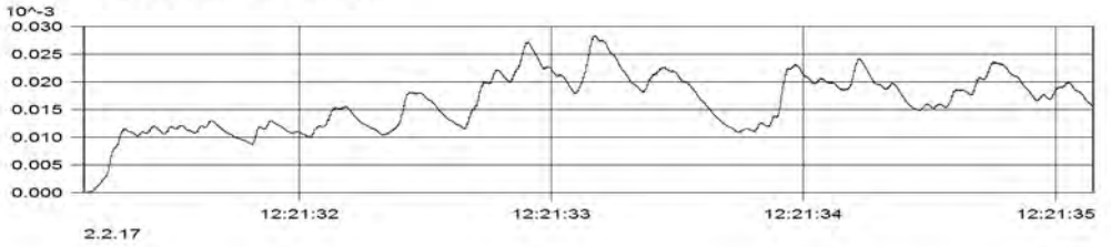
MP2.1 (Kanal_002) KB(max) = 0.028[-]
