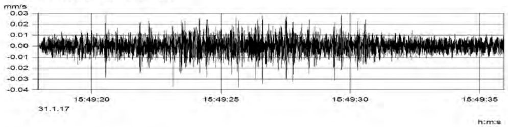
MP1 (Kanal_001) v(max) = 0.038 mm/s
