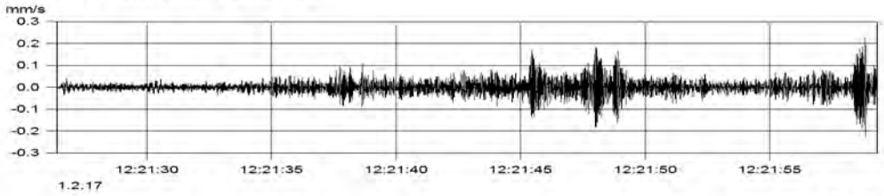
MP2.1 (Kanal_002) v(max) = 0.228 mm/s
