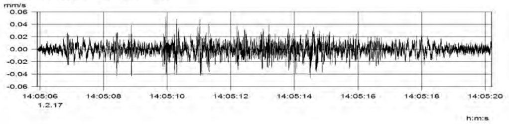
MP1 (Kanal_001) v(max) = 0.053 mm/s
