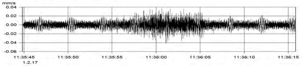
MP1 (Kanal_001) v(max) = 0.042 mm/s
