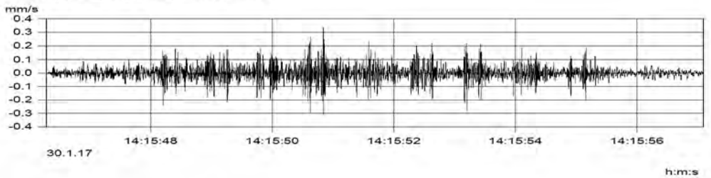
MP3.1 (Kanal_003) v(max) = 0.339 mm/s
