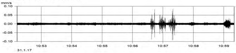
MP2 (Kanal_002) v(max) = 0.093 mm/s
