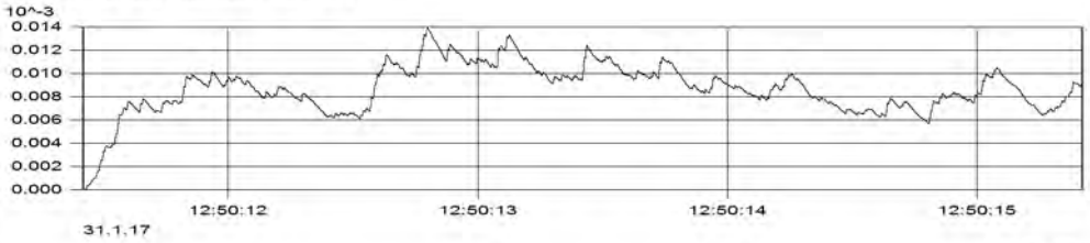
MP2 (Kanal_002) KB(max) = 0.014[-]
