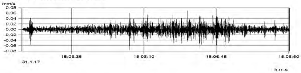
MP2.1 (Kanal_002) v(max) = 0.077 mm/s
