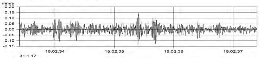
MP3.1 (Kanal_003) v(max) = 0.151 mm/s
