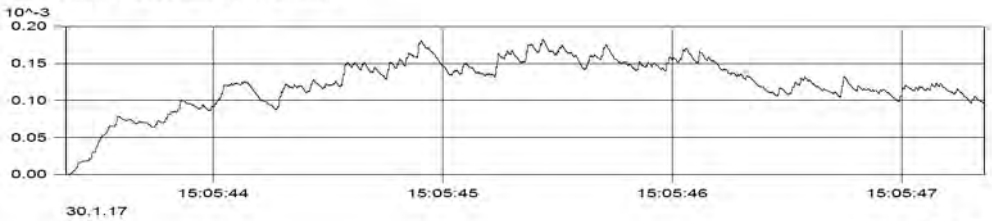
MP3.1 (Kanal_003) KB(max) = 0.183[-]
