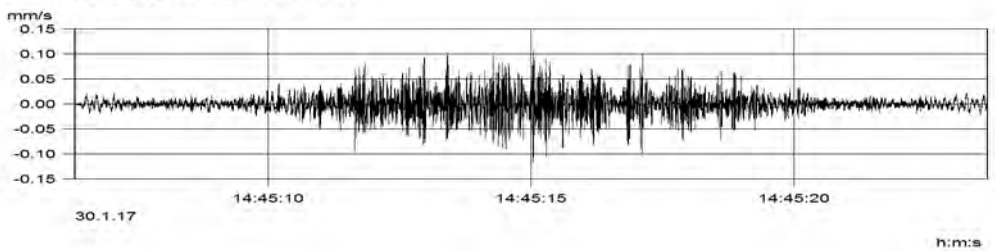
MP3.2 (Kanal_004) v(max) = 0.116 mm/s
