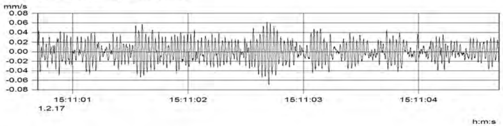
MP3.1 (Kanal_003) v(max) = 0.070 mm/s
