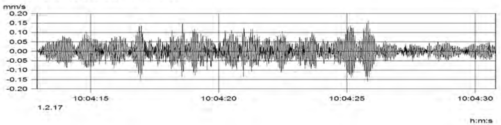
MP3.2 (Kanal_004) v(max) = 0.161 mm/s
