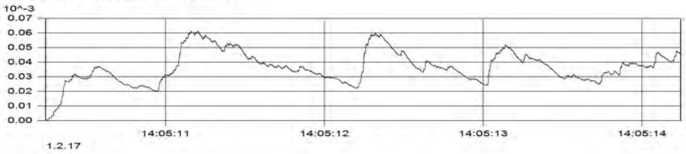
MP3.1 (Kanal_003) KB(max) = 0.061[-]
