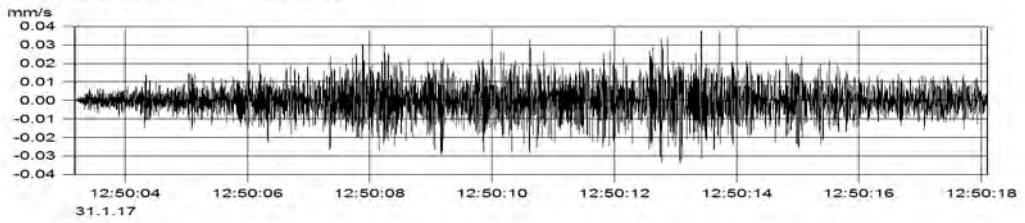
MP2 (Kanal_002) v(max) = 0.037 mm/s
