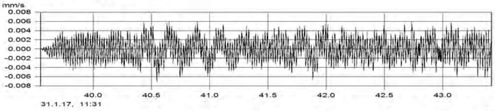
MP2 (Kanal_002) v(max) = 0.007 mm/s
