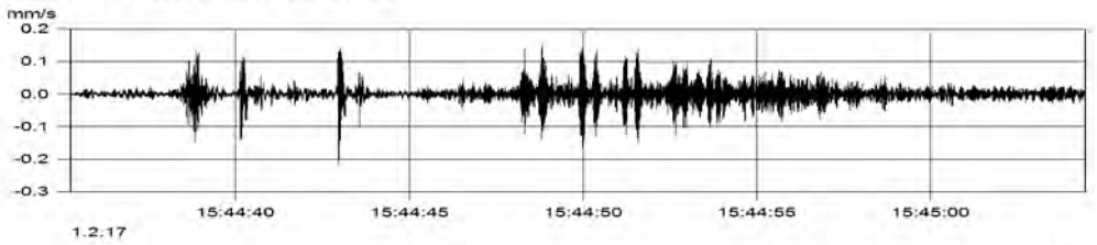
MP2.1 (Kanal_002) v(max) = 0.215 mm/s
