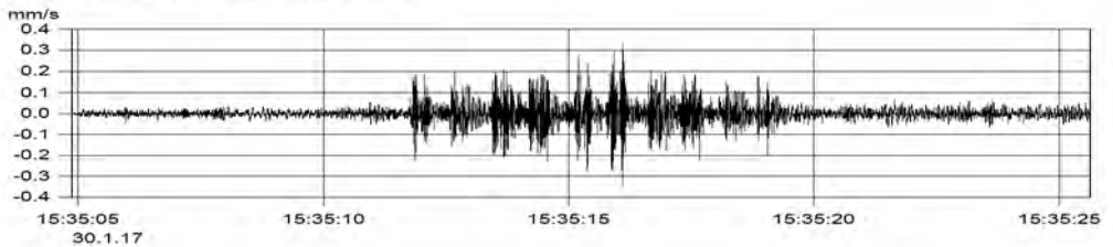
MP3.1 (Kanal_003) v(max) = 0.345 mm/s
