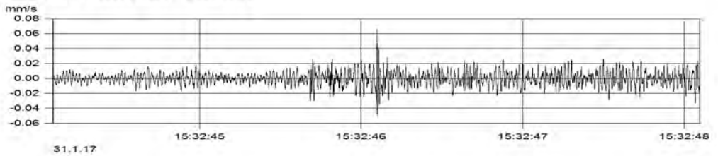
MP2.1 (Kanal_002) v(max) = 0.066 mm/s
