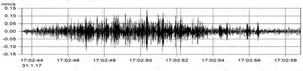
MP3.1 (Kanal_003) v(max) = 0.150 mm/s
