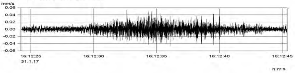
MP2.1 (Kanal_002) v(max) = 0.054 mm/s
