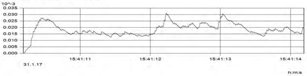
MP3.1 (Kanal_003) KB(max) = 0.031[-]
