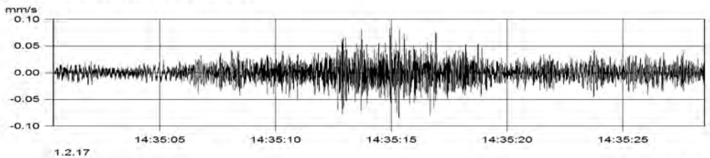
MP3.2 (Kanal_004) v(max) = 0.085 mm/s
