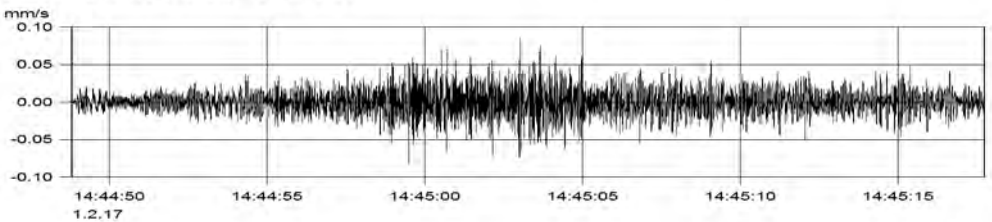
MP3.2 (Kanal_004) v(max) = 0.085 mm/s
