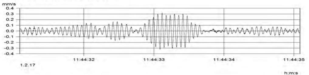
MP3.2 (Kanal_004) v(max) = 0.320 mm/s
