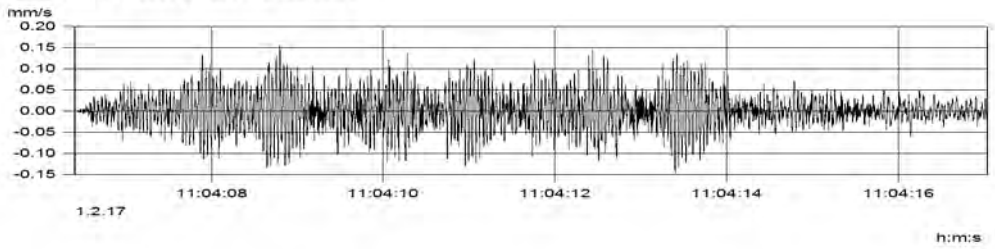
MP2.1 (Kanal_002) v(max) = 0.156 mm/s
