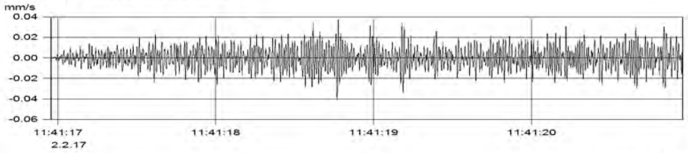
MP2.1 (Kanal_002) v(max) = 0.041 mm/s
