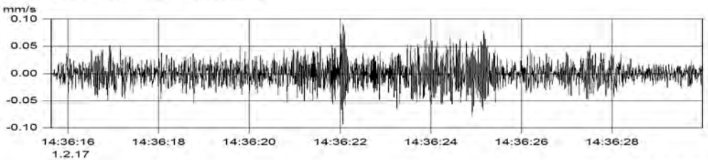
MP3.1 (Kanal_003) v(max) = 0.093 mm/s
