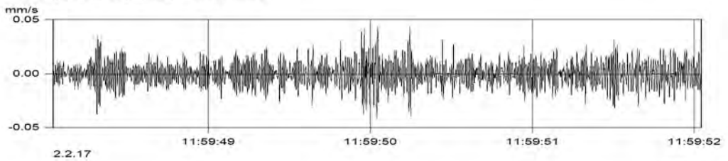
MP2.2 (Kanal_003) v(max) = 0.044 mm/s
