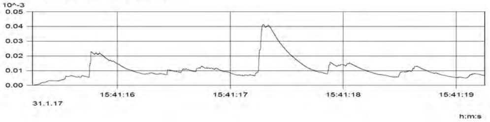
MP2.1 (Kanal_002) KB(max) = 0.041[-]
