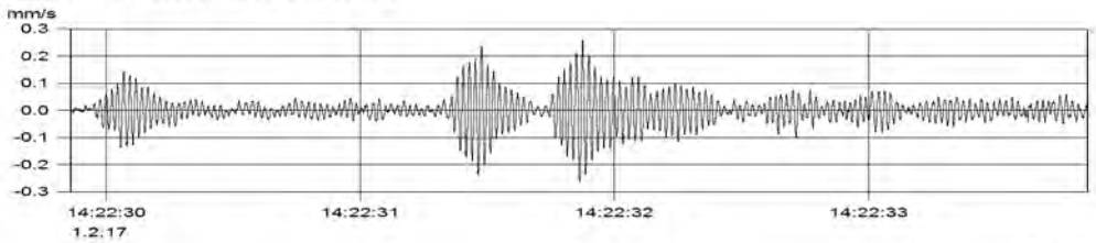
MP2.1 (Kanal_002) v(max) = 0.264 mm/s
