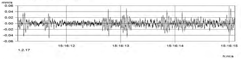
MP1 (Kanal_001) v(max) = 0.052 mm/s
