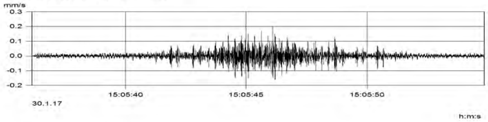
MP1 (Kanal_001) v(max) = 0.201 mm/s
