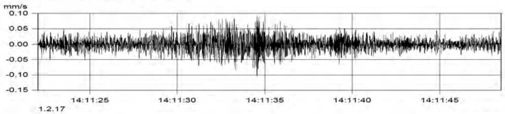
MP3.1 (Kanal_003) v(max) = 0.101 mm/s
