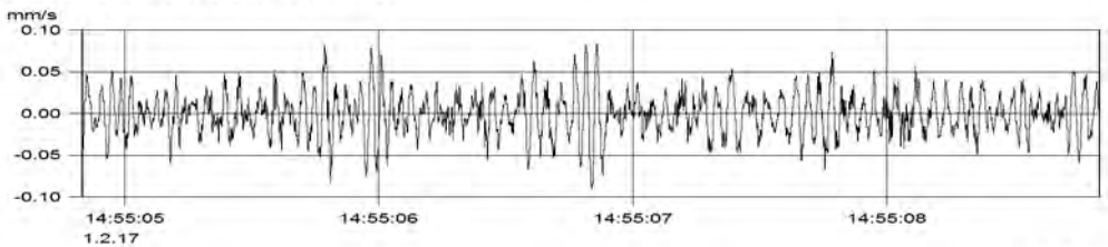
MP3.2 (Kanal_004) v(max) = 0.091 mm/s
