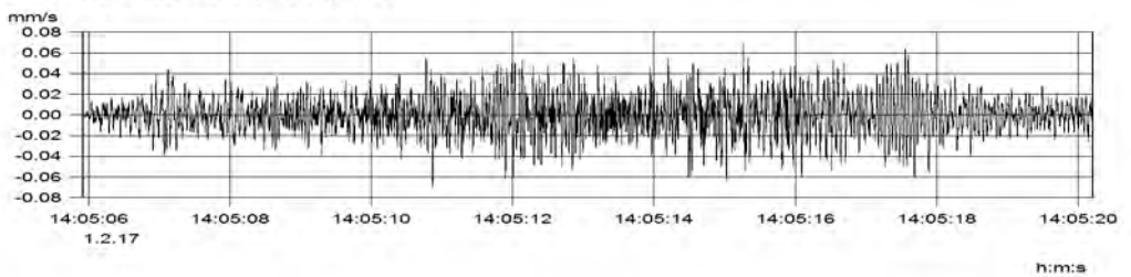
MP3.2 (Kanal_004) v(max) = 0.070 mm/s
