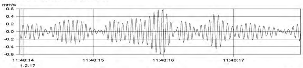
MP3.2 (Kanal_004) v(max) = 0.590 mm/s
