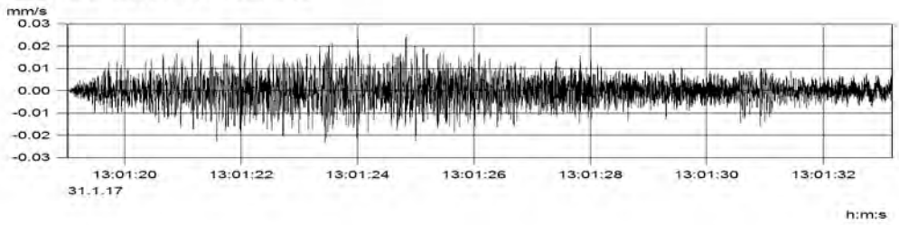
MP2 (Kanal_002) v(max) = 0.024 mm/s
