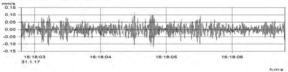
MP3.1 (Kanal_003) v(max) = 0.123 mm/s
