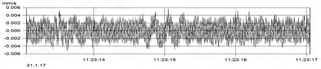
MP2 (Kanal_002) v(max) = 0.006 mm/s
