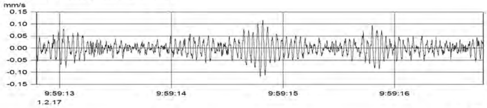
MP2.1 (Kanal_002) v(max) = 0.120 mm/s
