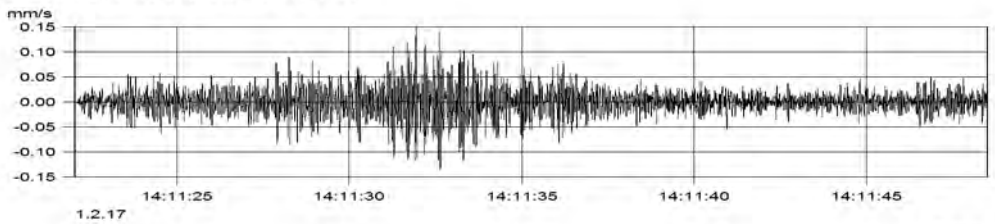
MP3.2 (Kanal_004) v(max) = 0.150 mm/s
