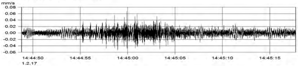
MP1 (Kanal_001) v(max) = 0.068 mm/s
