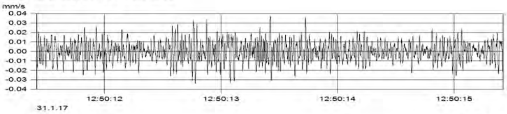
MP2 (Kanal_002) v(max) = 0.037 mm/s
