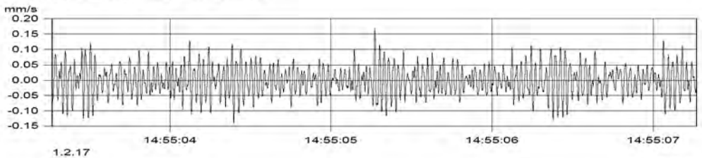
MP3.1 (Kanal_003) v(max) = 0.170 mm/s
