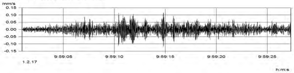
MP2.1 (Kanal_002) v(max) = 0.120 mm/s
