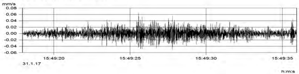
MP3.2 (Kanal_004) v(max) = 0.065 mm/s
