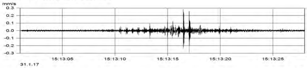
MP2.1 (Kanal_002) v(max) = 0.291 mm/s
