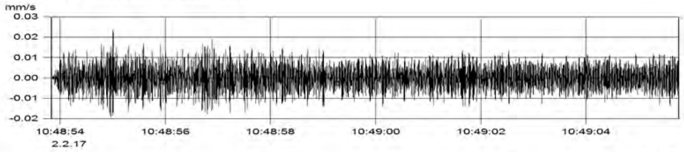
MP2.1 (Kanal_002) v(max) = 0.024 mm/s
