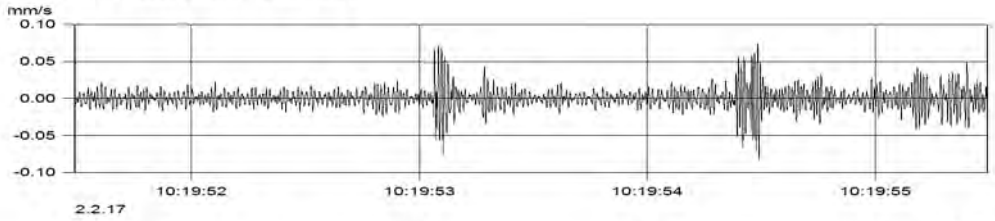
MP2.1 (Kanal_002) v(max) = 0.084 mm/s
