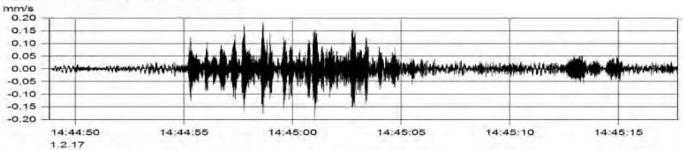
MP2.1 (Kanal_002) v(max) = 0.194 mm/s
