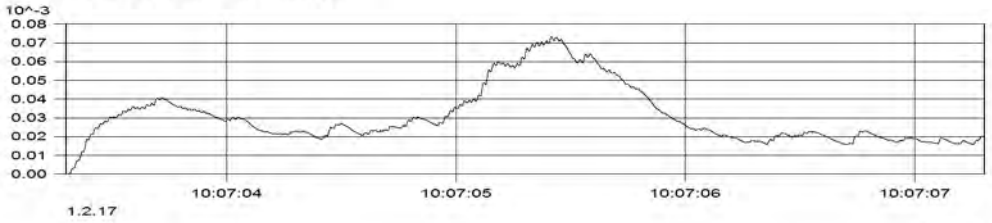
MP2.1 (Kanal_002) KB(max) = 0.073[-]
