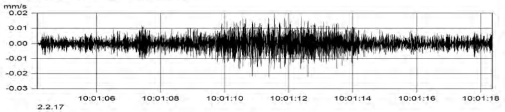
MP2.2 (Kanal_003) v(max) = 0.022 mm/s
