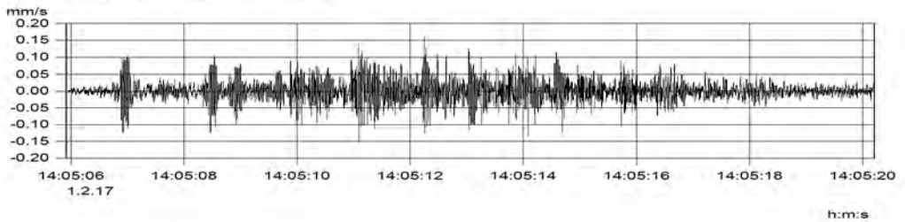
MP3.1 (Kanal_003) v(max) = 0.162 mm/s
