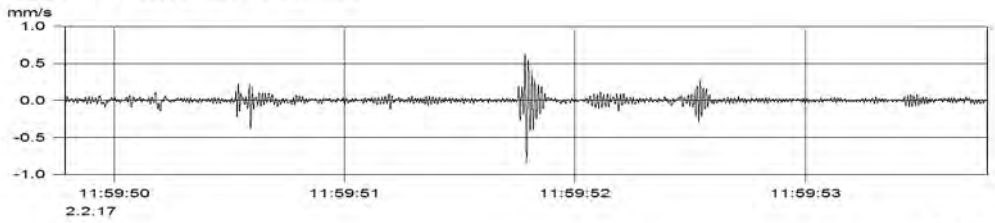
MP2.1 (Kanal_002) v(max) = 0.843 mm/s
