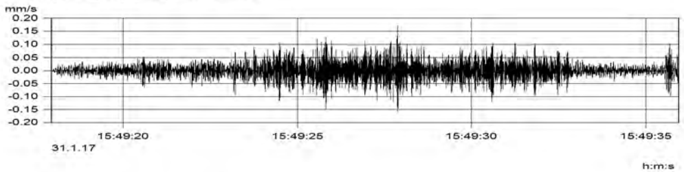
MP3.1 (Kanal_003) v(max) = 0.172 mm/s
