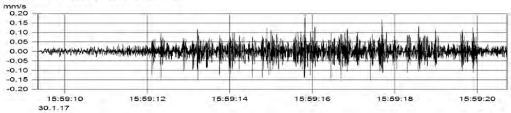
MP2.1 (Kanal_002) v(max) = 0.198 mm/s
