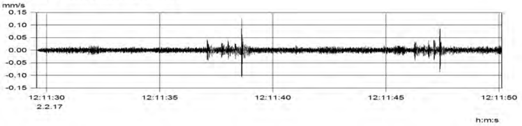
MP2.1 (Kanal_002) v(max) = 0.125 mm/s
