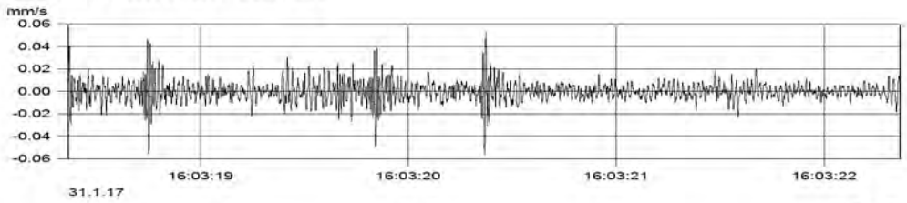
MP2.1 (Kanal_002) v(max) = 0.057 mm/s
