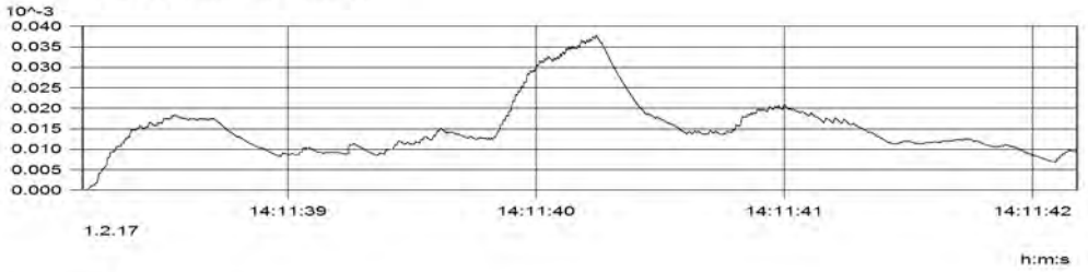
MP2.1 (Kanal_002) KB(max) = 0.038[-]
