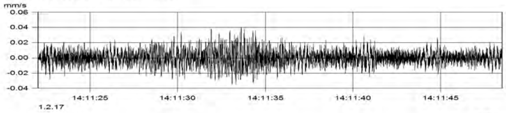
MP1 (Kanal_001) v(max) = 0.041 mm/s
