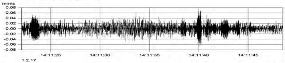
MP2.1 (Kanal_002) v(max) = 0.068 mm/s
