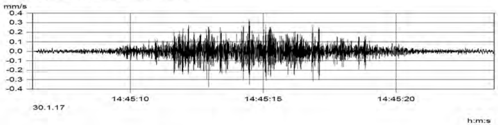
MP3.1 (Kanal_003) v(max) = 0.377 mm/s
