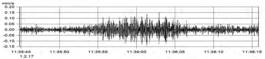
MP3.1 (Kanal_003) v(max) = 0.155 mm/s
