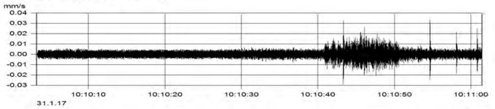
MP2 (Kanal_002) v(max) = 0.033 mm/s
