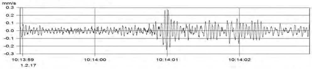
MP2.1 (Kanal_002) v(max) = 0.269 mm/s
