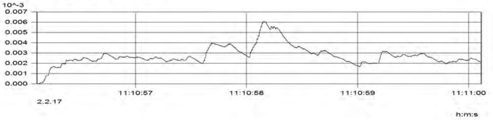
MP2.2 (Kanal_003) KB(max) = 0.006[-]
