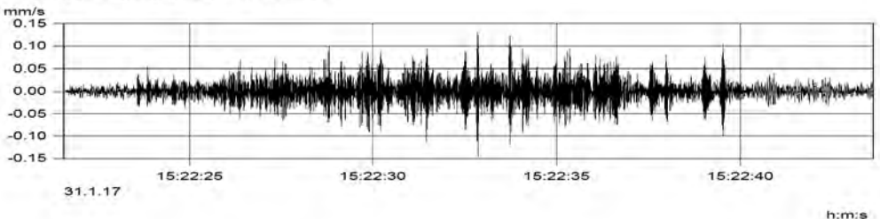
MP3.1 (Kanal_003) v(max) = 0.146 mm/s
