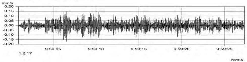
MP3.1 (Kanal_003) v(max) = 0.174 mm/s
