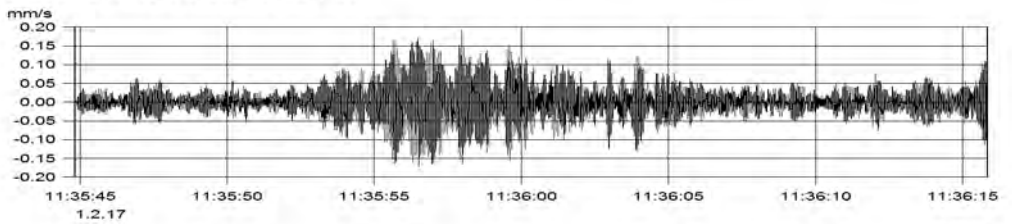
MP3.2 (Kanal_004) v(max) = 0.192 mm/s
