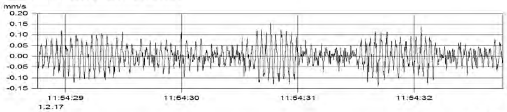
MP2.1 (Kanal_002) v(max) = 0.153 mm/s
