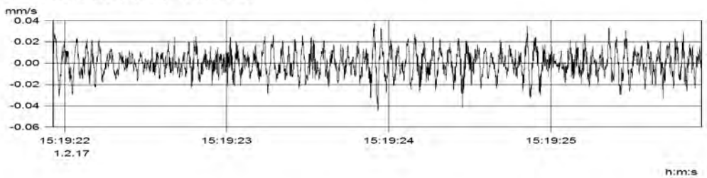
MP3.2 (Kanal_004) v(max) = 0.045 mm/s
