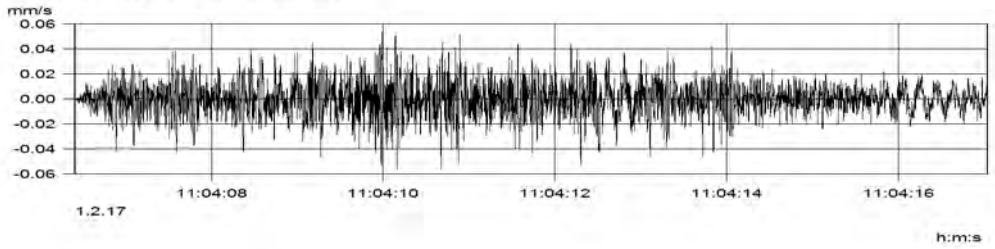
MP1 (Kanal_001) v(max) = 0.056 mm/s
