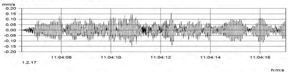
MP3.2 (Kanal_004) v(max) = 0.157 mm/s
