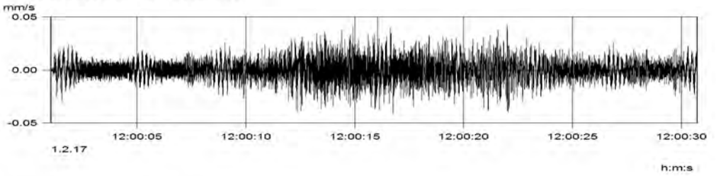
MP1 (Kanal_001) v(max) = 0.050 mm/s
