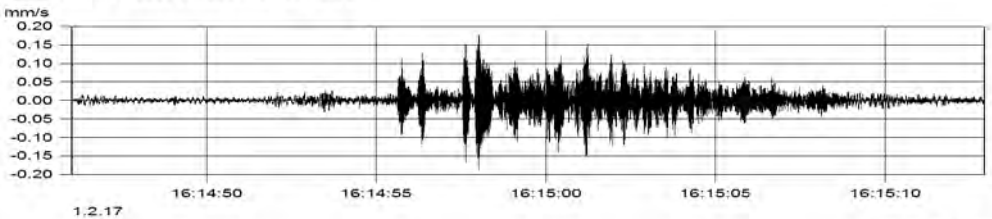
MP2.1 (Kanal_002) v(max) = 0.187 mm/s
