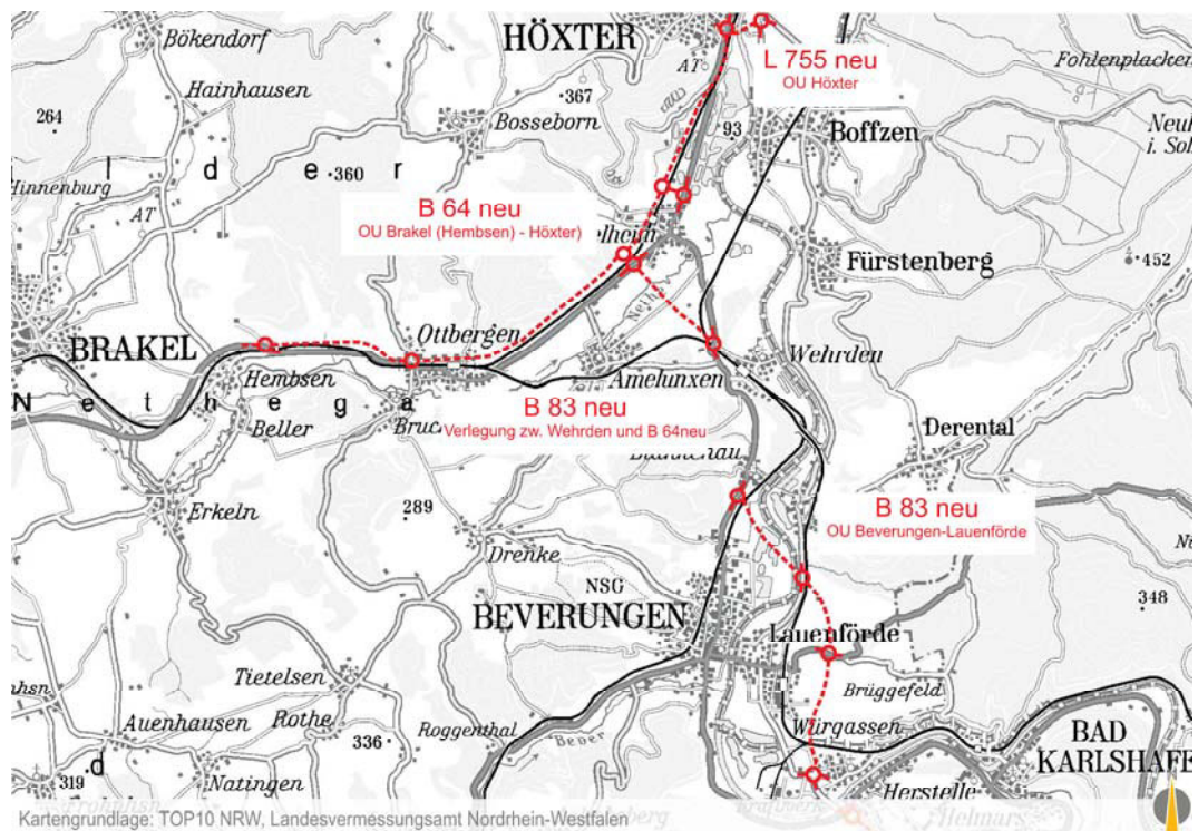
Abbildung 4 Übersichtsplan Planungsfall 1
