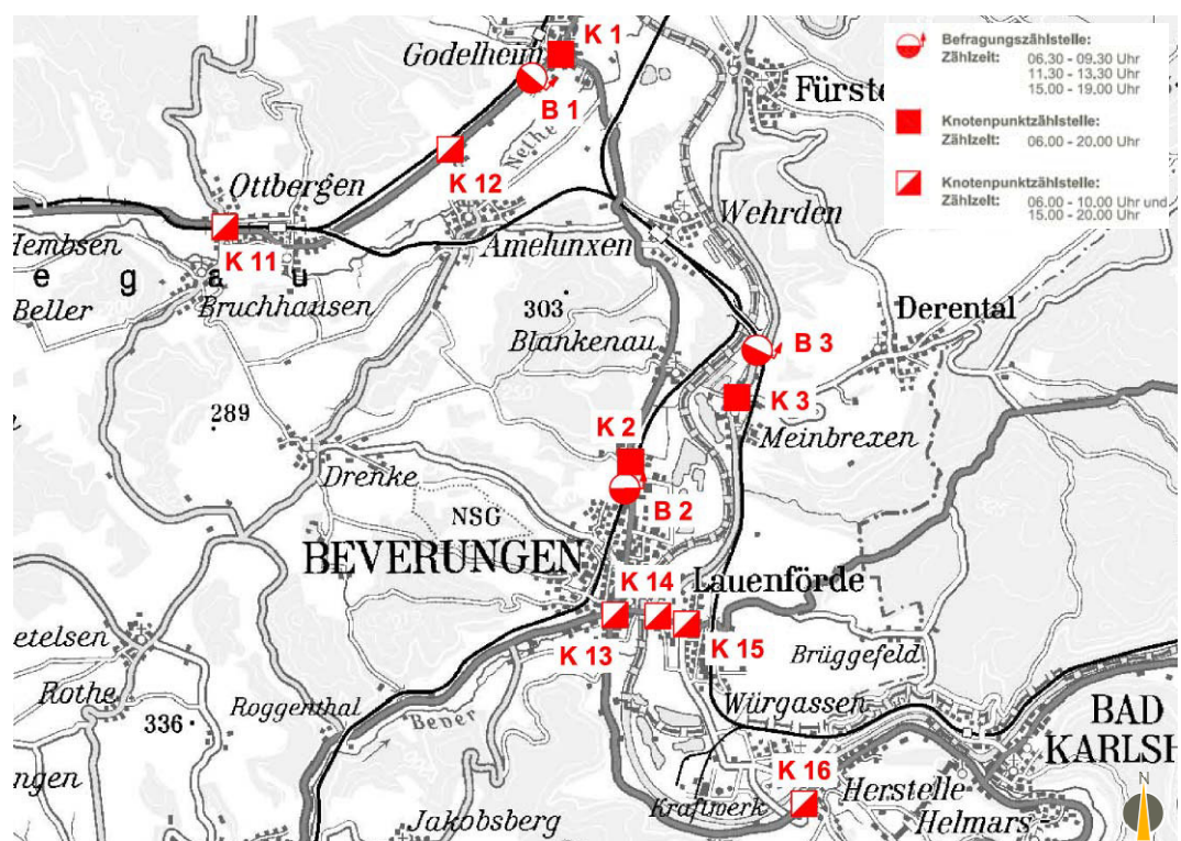
Abbildung 2 Übersichtplan Verkehrserhebung
