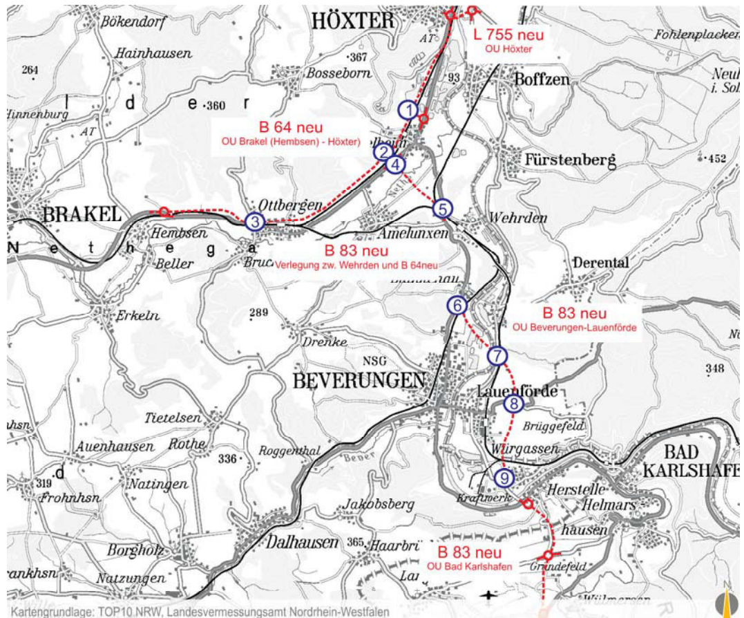
Abbildung 5 Übersichtsplan Knotenpunkte
