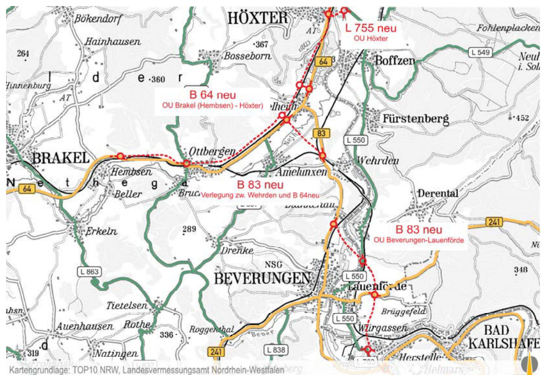
Abbildung 1 Übersichtsplan Verkehrsuntersuchung
