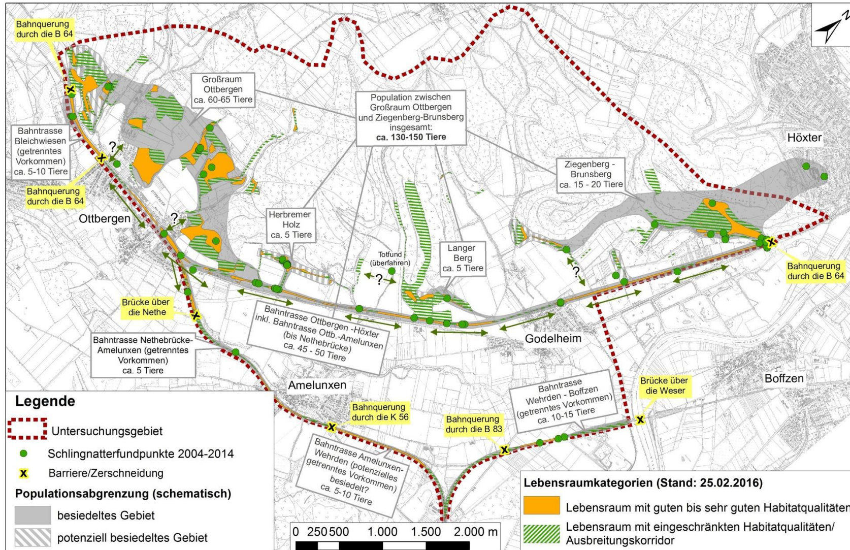
Abbildung 10: Verbreitung der Schlingnatter im Untersuchungsgebiet (inkl. Populationsabgrenzung und Bestandsschätzung; schematische Darstellung).
