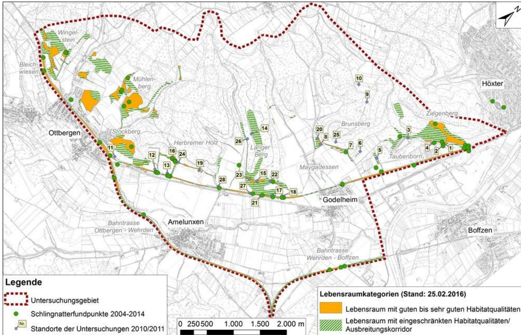
Abbildung 5: Potenziell geeignete Lebensräume für die Schlingnatter ( Coronella austriaca ) im Untersuchungsgebiet.
