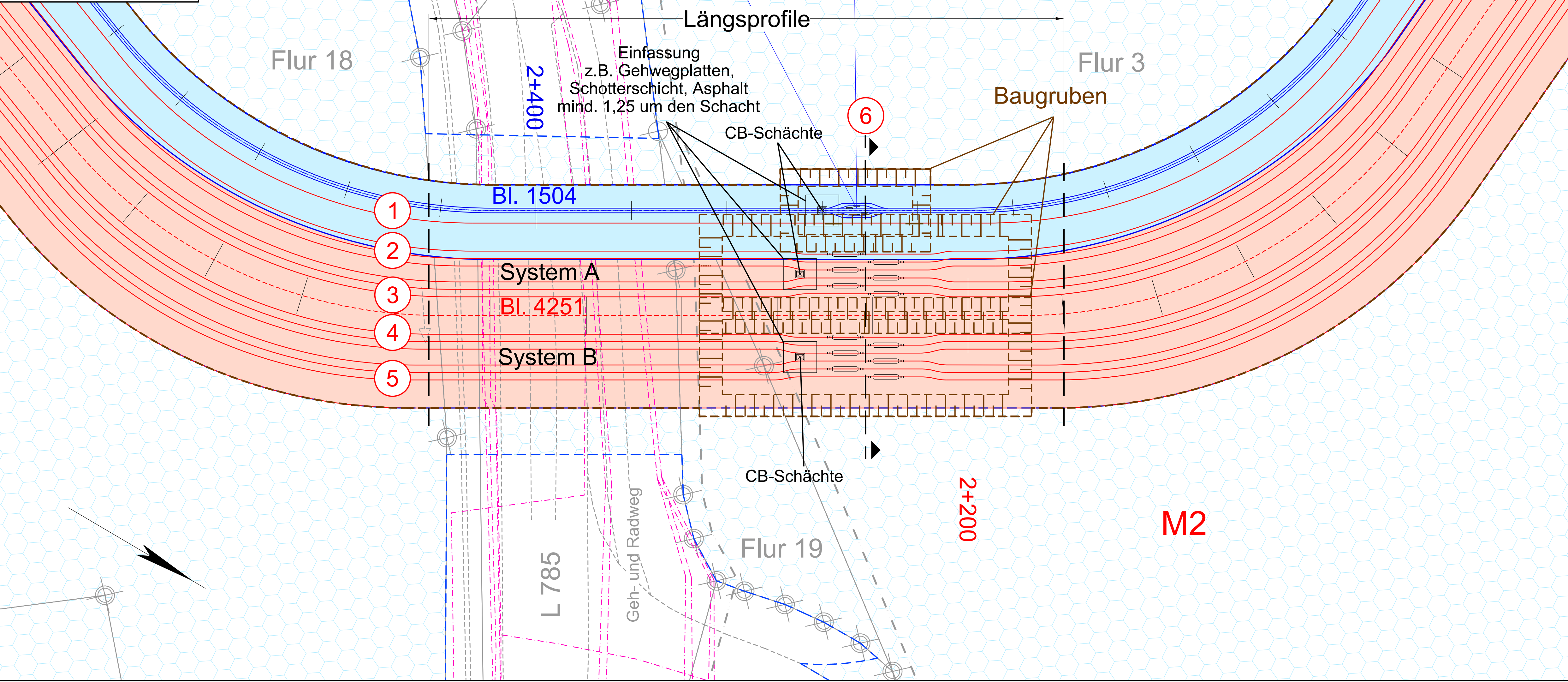
Lageplan Maßstab 1: 250
